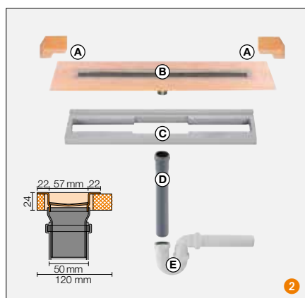
Guarnição Schlüter-KERDI, horizontal para montagem ao centro
