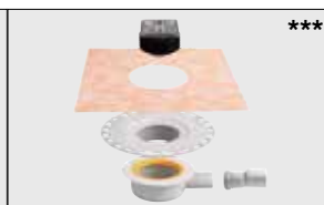
Schlüter®-KERDI-DRAIN-BASE 1 conjunto (com grelha decorativa 1)
