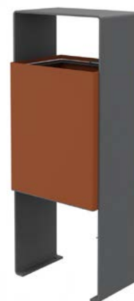
Ecoponto 8 Recycle Bin 8 13125 60 Lt 42x31x106 cm \approx 65 kg Aparafusamento de Superfície Surface Bolted Anchoring
