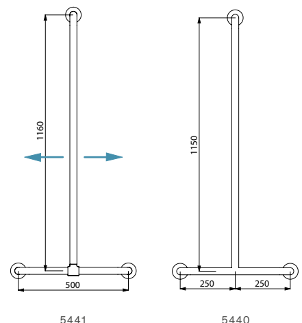
Colocação da barra vertical (ref. 5441)
