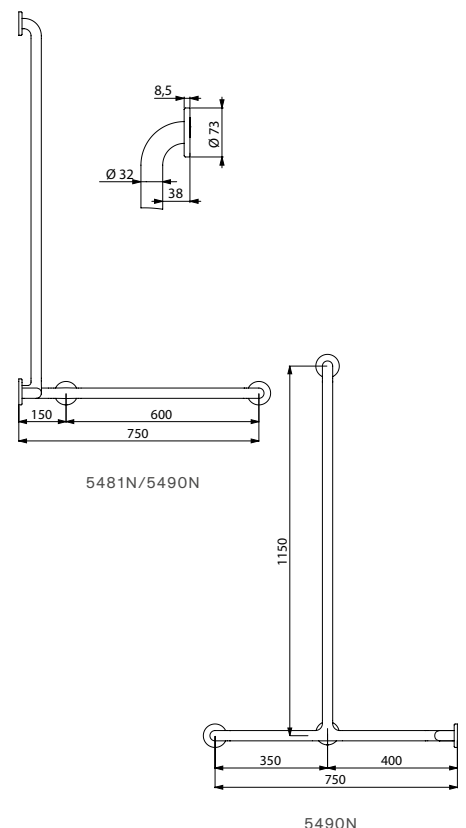
Colocação da barra vertical regulável à esquerda ou à direita (ref. 5481N)
