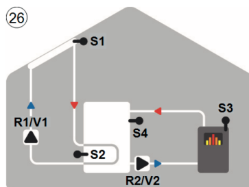
26 Solar com armazenamento e caldeira de combustível sólido e S4
