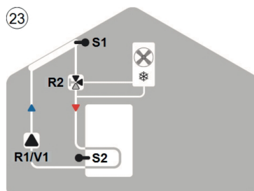
23 Solar com arrefecimento de 1 (coletor de arrefecimento)
