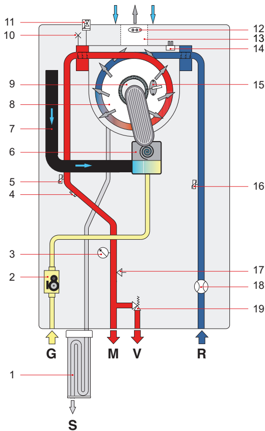
ITACA CH | KR 45 60 85 120 150 | esquema hidráulico
