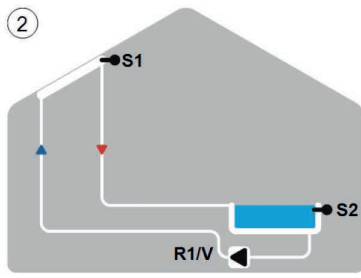
Solar com piscina
