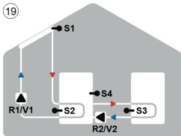
19 Solar com armazenamento de transferência
