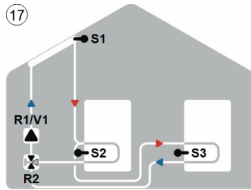
17 Solar com 2 depósitos e válvula de comutação
