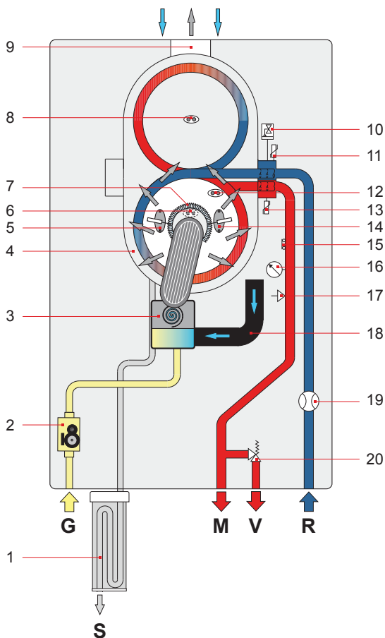
ITACA CH | KR 45 60 85 120 150 | esquema hidráulico
