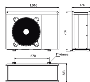
Unidade exterior 7 kW
