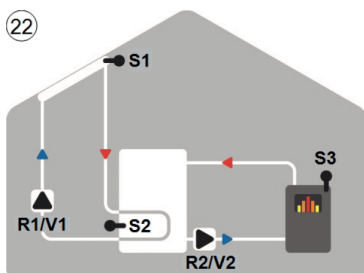
22 Solar e caldeira de combustível sólido
