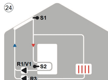
24 Solar com arrefecimento de 2
