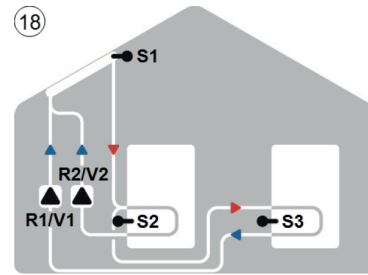
18 Solar com 2 depósitos e bombas 2
