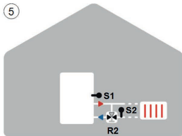
Aumento do fluxo de retorno do circuito de aquecimento
