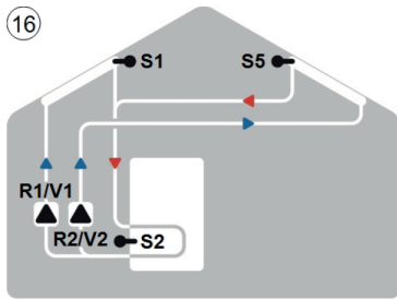
16 Solar com 2 coletor de superfícies e 2 bombas
