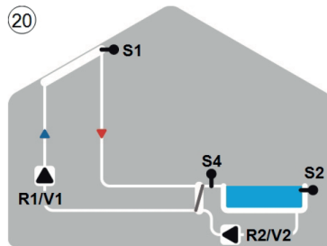
20 Solar com piscina e permutador de calor
