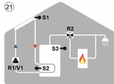
21 Solar com termostato e válvula
