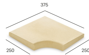
3 375 x 375 x 30 - 50 mm canto interno raio 150 radius 150 internal corner
