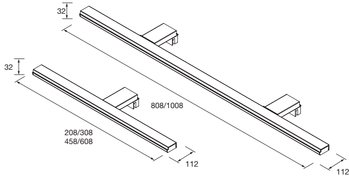
Aplique PANDORA 208 cromado brilho luz led (5 W- 5700°K). IP 44 fixação multiencaixe 208 x 112 x 32 mm 24548 63 € Aplique PANDORA 308 cromado brilho luz led (8 W- 5700°K). IP 44 fixação multiencaixe 308 x 112 x 32 mm 21735 78 € Aplique PANDORA 458 cromado brilho luz led (1x10 W- 5700°K). IP 44 fixação multiencaixe 458 x 112 x 32 mm 23534 105 € Aplique PANDORA 608 cromado brilho luz led (1 x 11 W- 5700°K). IP 44 fixação multiencaixe 608 x 112 x 32 mm 23535 126 € Aplique PANDORA 800 cromado brilho luz led (1 x 15 W -5700°K). IP 44 fixação multiencaixe 808 x 112 x 32 mm 23536 170 € Aplique PANDORA 1008 cromado brilho luz led (1 x 15 W -5700°K). IP 44 fixação multiencaixe 1008 x 112 x 32 mm 24549 204 €
