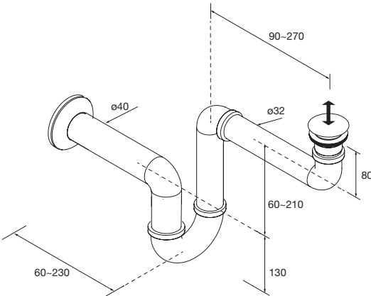
Jogo de sifão reduzido com válvula descarga clic-clac 19366 69 €
