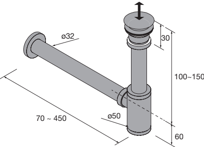
Sifão VINCI Preto mate com válvula click 26985 124 €
