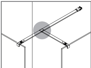
Conector para dois suportes
