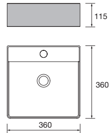
new product Lavatório de pousar TALEA Solid surface Bicolor sem sifão nem válvula clic-clac 360 x 115 x 360 mm 97652 315 €
