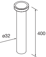
Tubo complementar Cromado de altura para qualquer sifão Ø32 x 400 mm 7787 26 €
