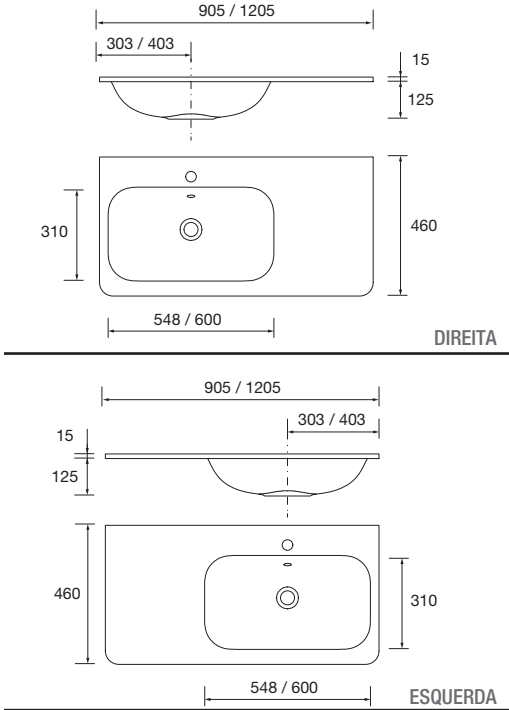
Lavatório UNIQ 905 coqueta à esquerda Mineralsolid mate sem sifão nem válvula clic-clac 905 x 15 x 460 mm 24544 425 €
