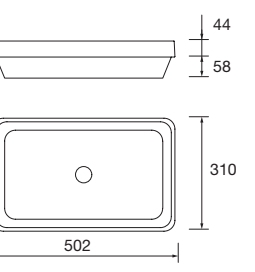
new product Lavatórios semiembutidos MAEL Solid surface Bicolor sem sifão nem válvula clic-clac 502 x 44 x 310 mm 97655 315 €
