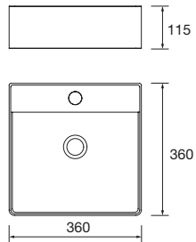
new product Lavatório de pousar TALEA Solid surface branco mate sem sifão nem válvula clic-clac 360 x 115 x 360 mm 97649 295 €
