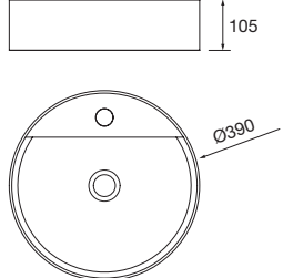
new product Lavatório de pousar BICA Solid surface Bicolor sem sifão nem válvula clic-clac Ø 390 x 105 mm 97648 315 €
