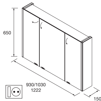
Armário ALLIANCE 1200 3 portas espelho duplo com interruptor e tomada e luz led lateral, IP44 (21,5W) 1222 x 650 x 150 mm 83166 1063 €
