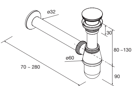
Sifão com válvula aberta de descarga Latão cromado 16994 75 €
