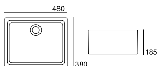
Pia Sintra . Piła Sintra . Sintra Sink . Évier Sintra 78615XX2C
