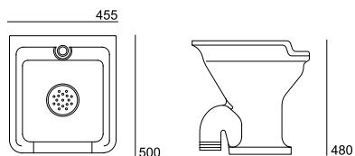
Pia hospitalar . Piła vertedero . Medical slop hooper . Évier d'hôpital 18613XX2K
