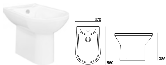
Bidé . Bidet 13411XX2K
