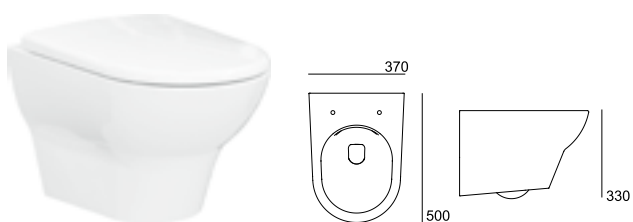
Sanita . Inodoro . Toilet . Toilette 42501XX2K
