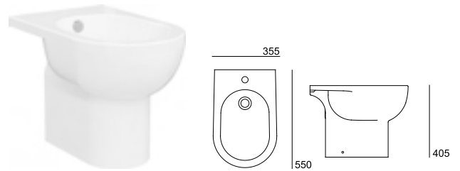
Bidé . Bidet 37411XX2K
