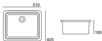
Pia Silves . Piła Silves . Silves Sink . Évier Silves 78616XX2C
