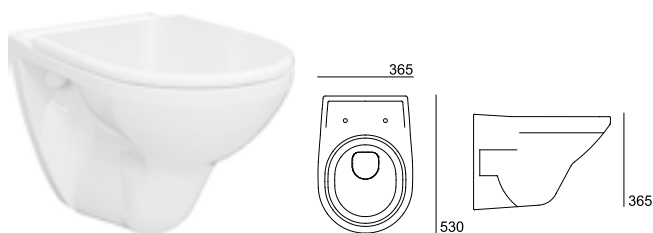
Sanita . Inodoro . Toilet . Toilette 13002XX2K
